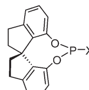
2a X = OR 2b X = NR 2 , SIPHOS
